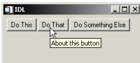
Figure 23-1: A Tooltip
